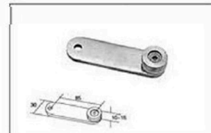
TK-1409
